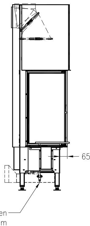
Seitenansicht M~1:20
