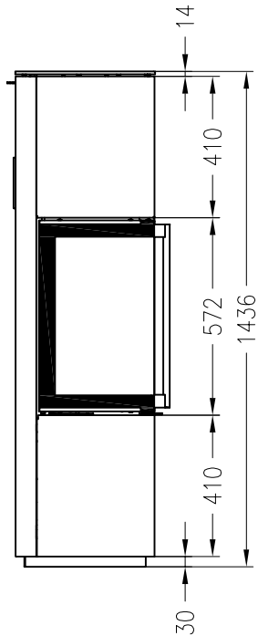
Seitenansicht M~1:20
