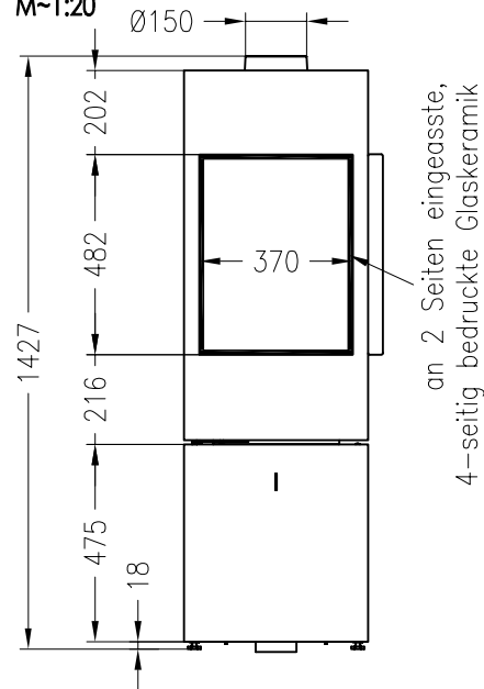
Vorderansicht M~1:20
