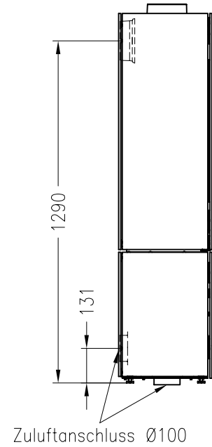
Seitenansicht von links M~1:20
